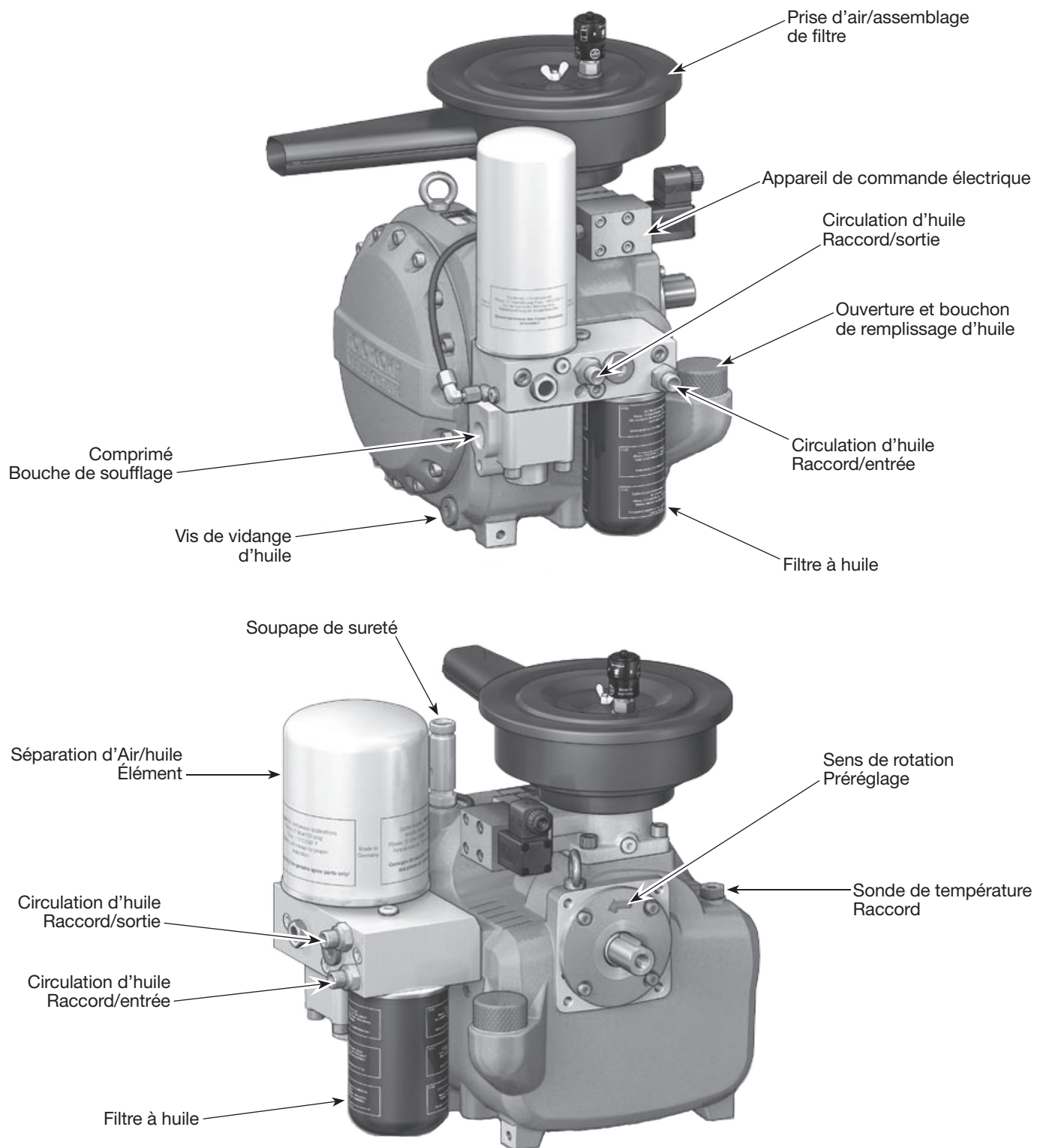
Figure 3 - Composants de l'extrémité air
