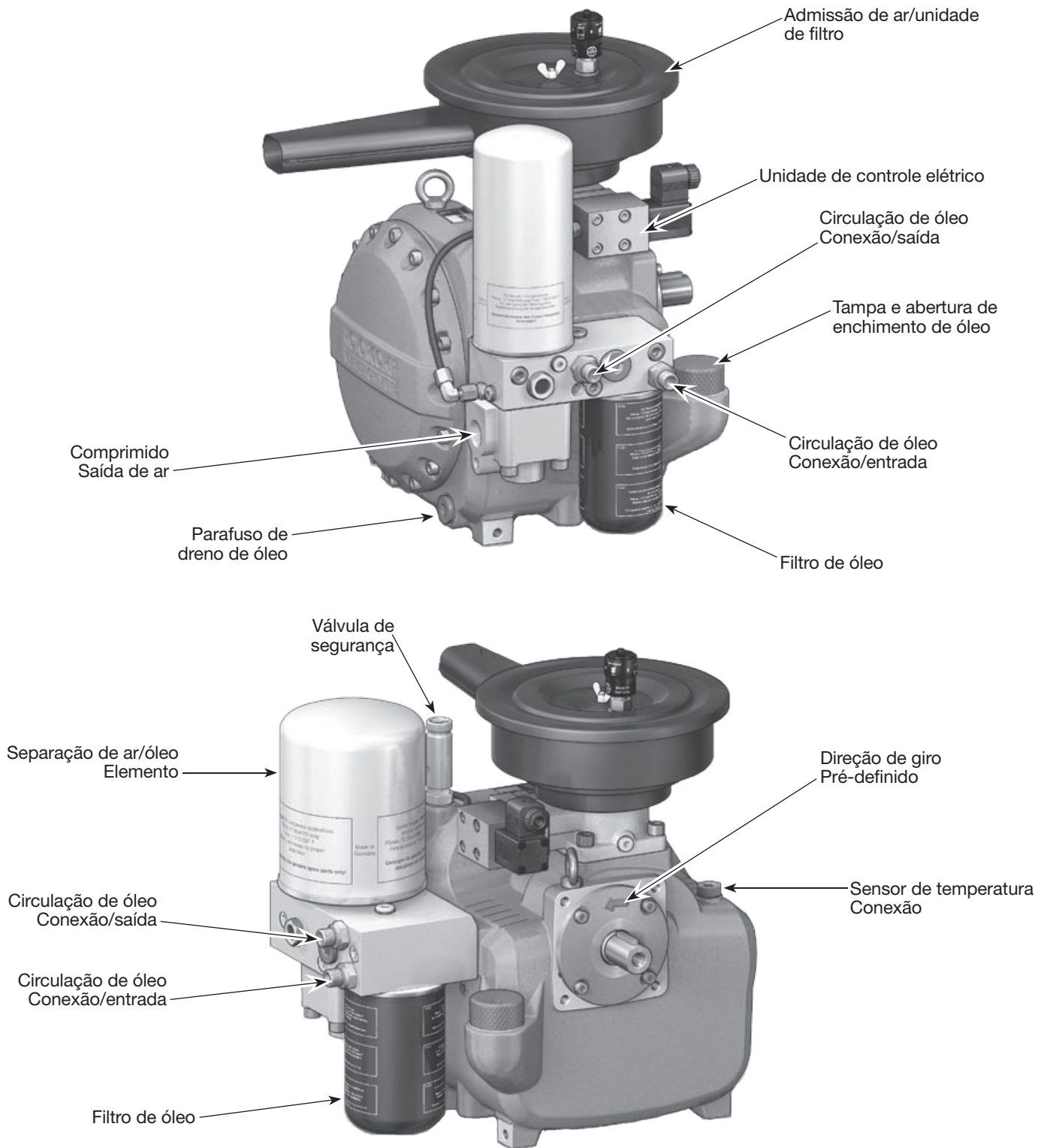
Figura 3 - Componentes da extremidade de ar
