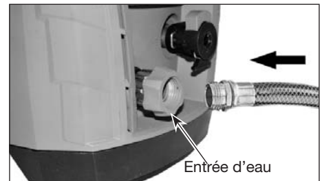
Figure 9 - Attachez le tuyau d'arrosage à l'unité
