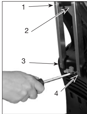
Figure 4 - Deslice la manija hacia la unidad (PW182501)
