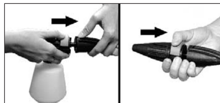
Figure 7- Conecte la lanza a la pistola o botella de detergente
