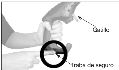
Figura 10 - Pasador de seguridad del gatillo
