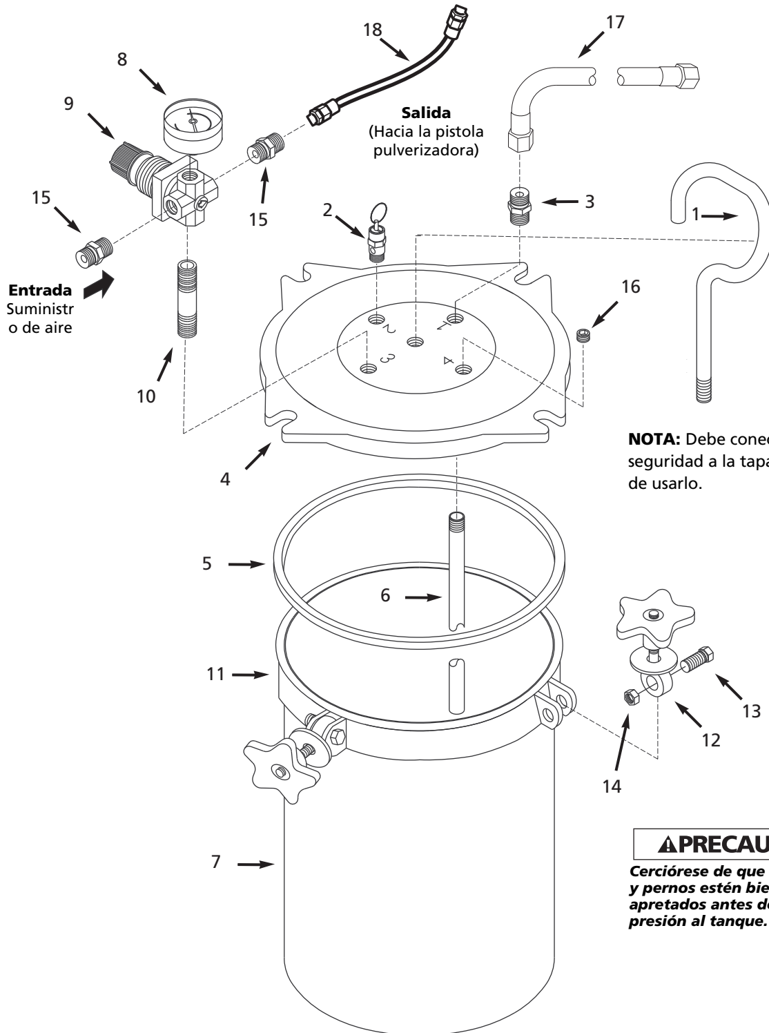
Figura 7 — Ilustración de los Repuestos
