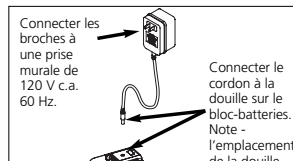
Figure 3 Charger le bloc-batteries - tous les modèles.
