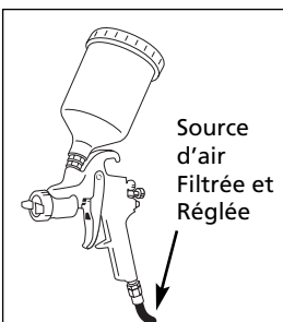
Figure 2 - Montage du Godet - Alimentation À Gravité
