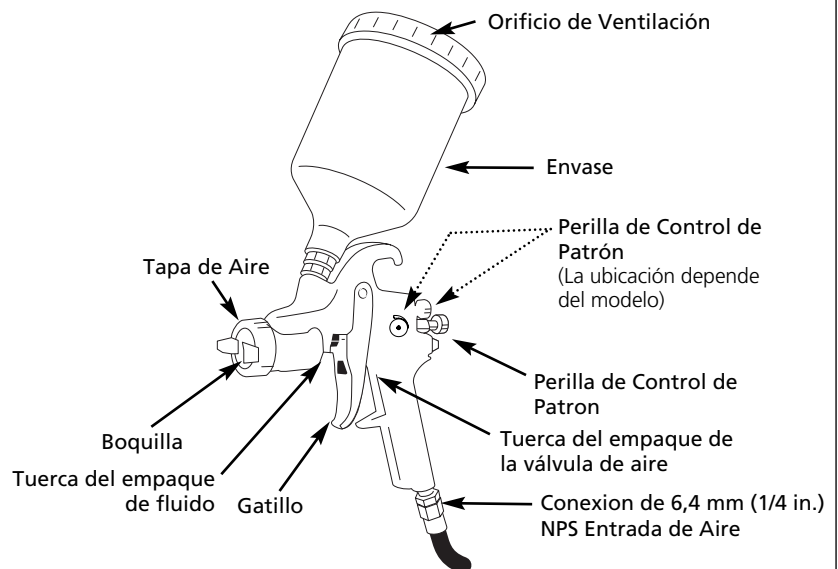
Figura 5 - Pistola Pulverizadora con Sistema de Alimentación de Gravedad
