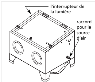
Figure 3 – Cabine de décapage de table
