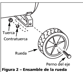
Figura 2 – Ensamble de la rueda
