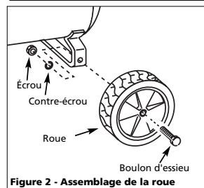
Figure 2 - Assemblage de la roue
