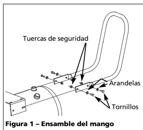
Figura 1 – Ensamble del mango
