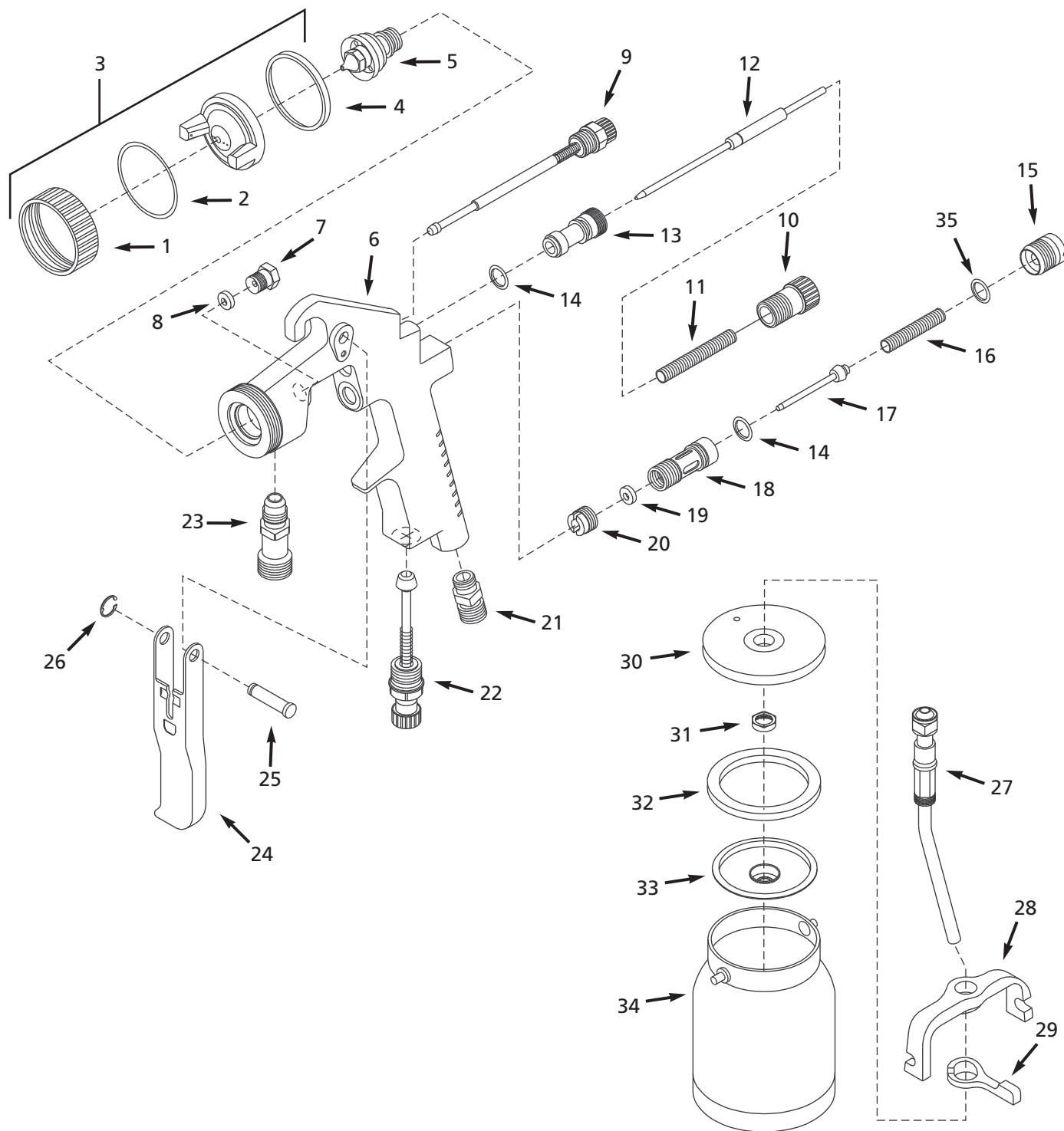
Figura 2 – Ilustración de las Partes de Reparación
