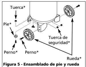
Figura 5 - Ensamblado de pie y rueda
