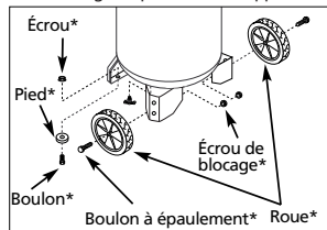
Figure 5 - Montage de Pied et de Roues
