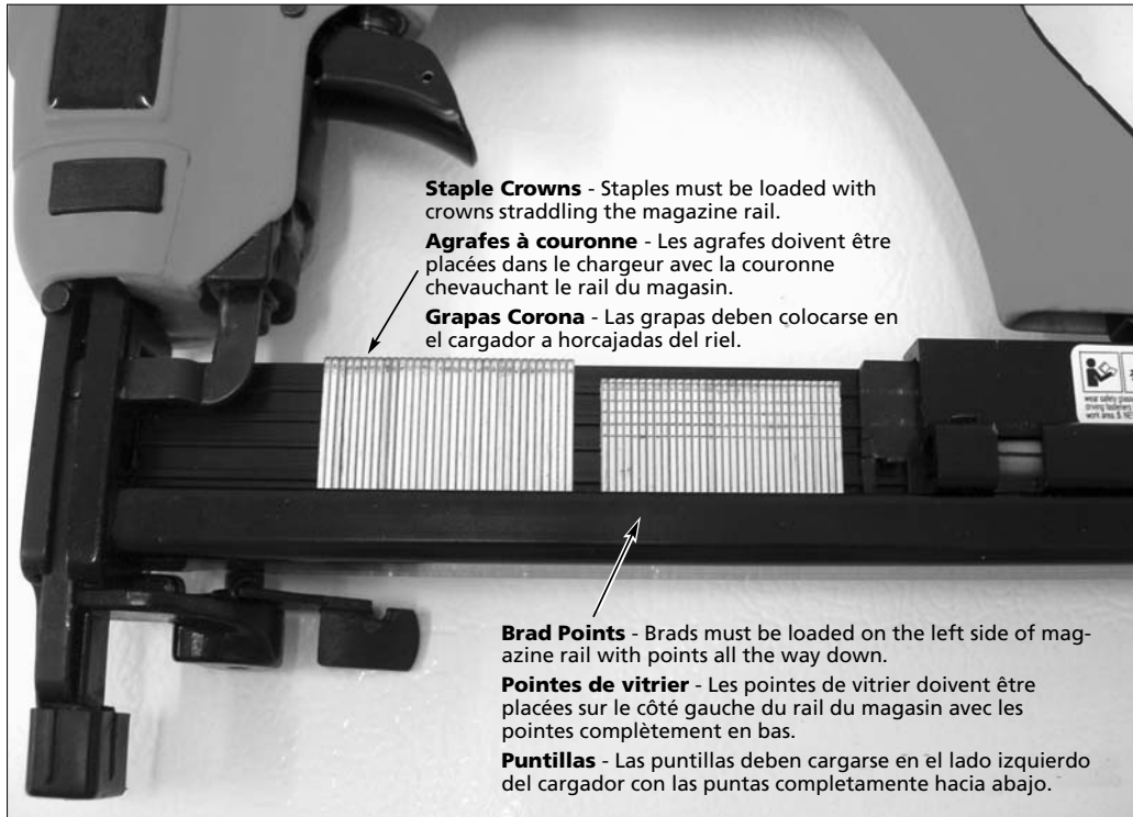
Figure 1 - Proper fastener placement in the 2-in-1 tool magazine Figure 1 - Placement correct des attaches dans le chargeur de l'outil 2-en-1 Figura 1 - Colocación correcta del sujetador en el cargador de la herramienta 2-en-1
