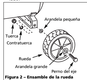
Figura 2 - Ensamble de la rueda
