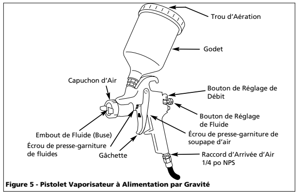
Figure 5 - Pistoleto Vaporizzatore a Alimentazione per Gravità
