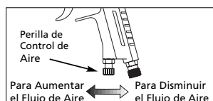
Figura 4 - Para Ajustar el Suministro de Aire a la Pistola Pulverizadora
