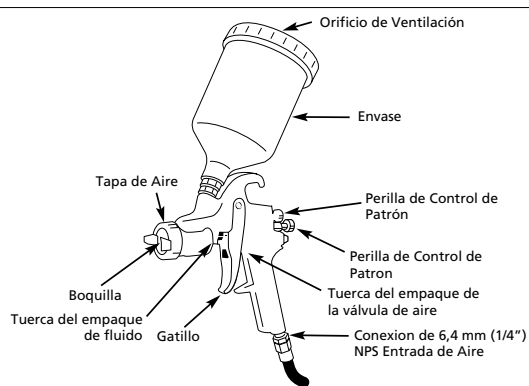
Figura 5 - Pistola Pulverizadora con Sistema de Alimentación de Gravedad
