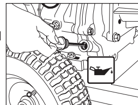
Figura 3 - Añadir/verificar aceite
